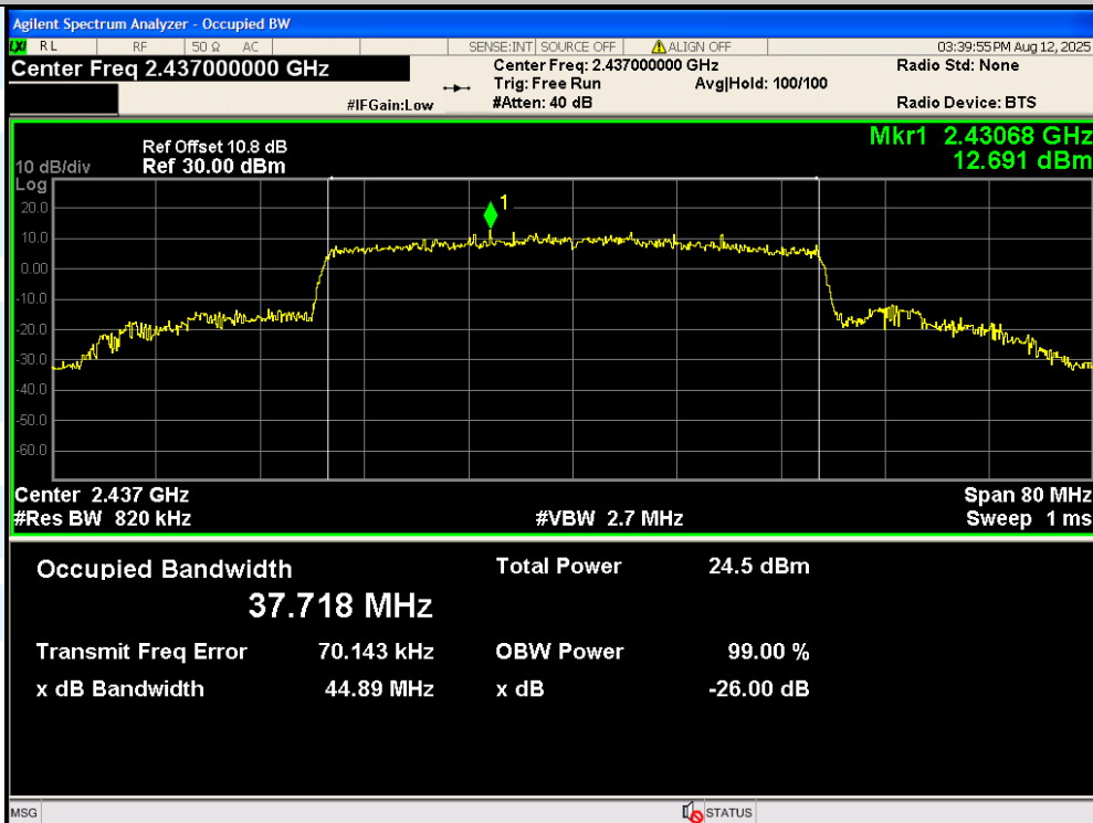
11AX40MIMO-Ant2-2437
