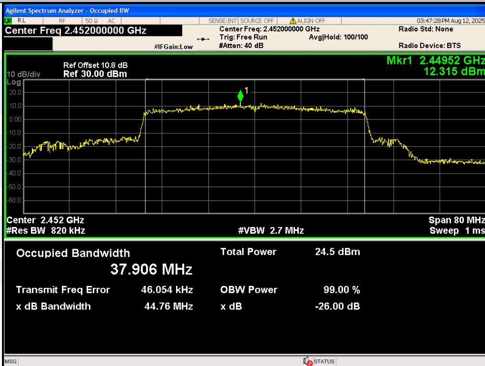
11AX40MIMO-Ant2-2452
