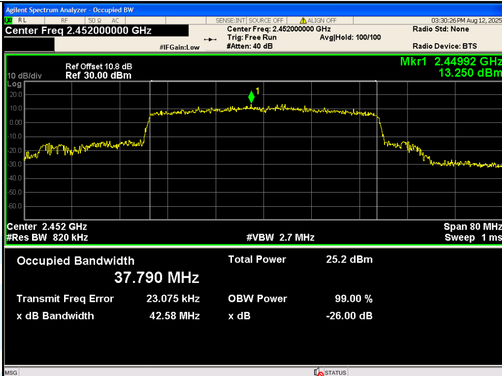
11AX40MIMO-Ant1-2452
