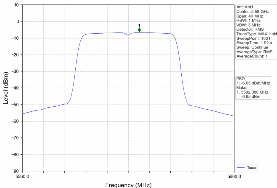
802.11n(HT20)_MCH_5580MHz_Ant1_NTNV
