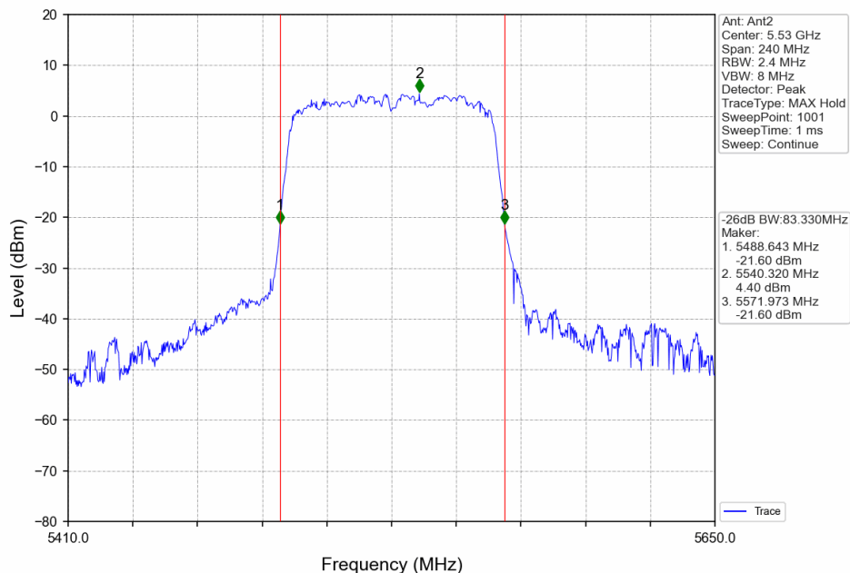
802.11ac(VHT80)_LCH_5530MHz_Ant2_NTNV
