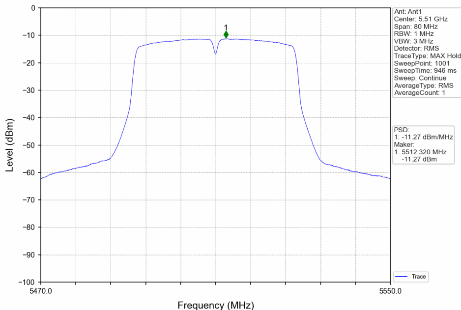
802.11n(HT40)_LCH_5510MHz_Ant1_NTNV
