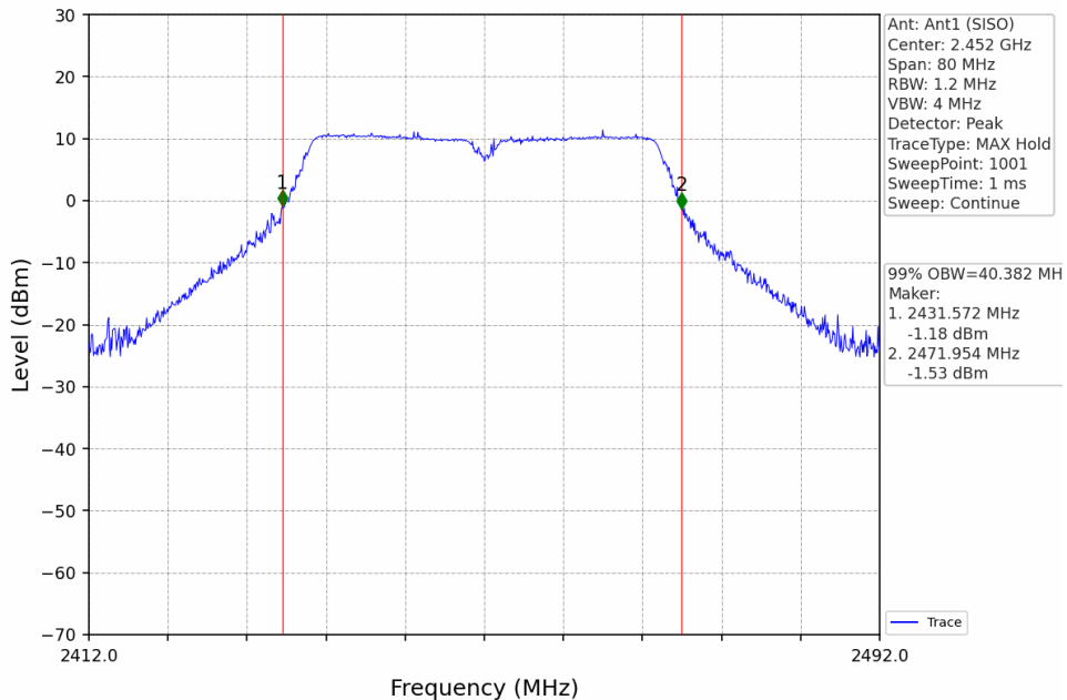
802.11n(HT40) HCH 2452MHz Ant1 (SISO) NTNV
