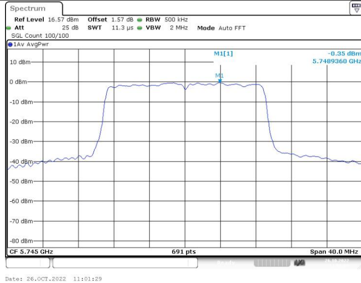
11AC20MIMO_Ant2_5745
