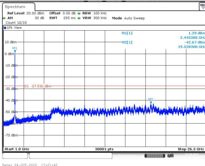
11N40MIMO_Ant2_2437_0~Reference
