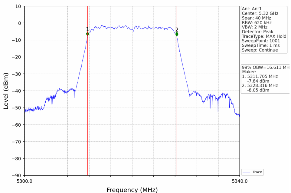
802.11n(HT20)_HCH_5320MHz_Ant1_NTNV
