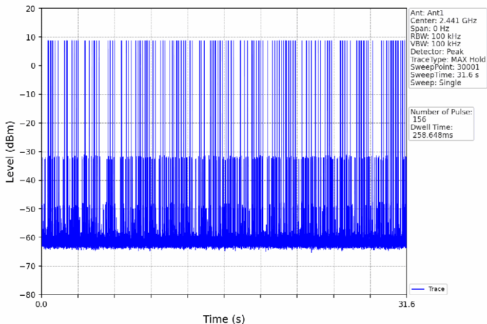
8DPSK_3DH3_HOPP_Ant1_NTNV
