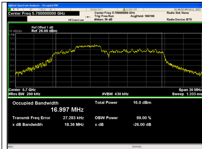
IEEE 802.11ax_Channel 140_20MHz_Antenna 0_RU&Index 52RU38
