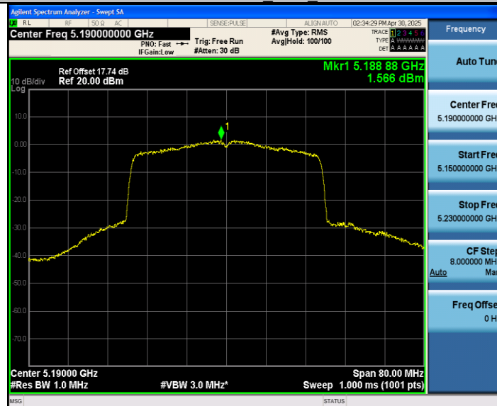
11AX40MIMO_Ant2_5190
