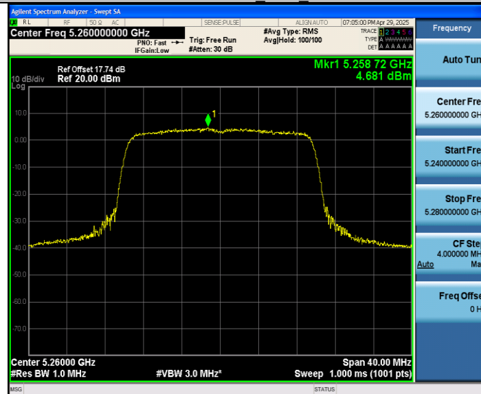
11AX20MIMO_Ant2_5260
