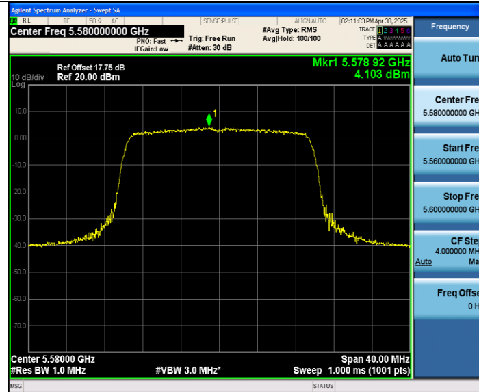
11AX20MIMO_Ant2_5580
