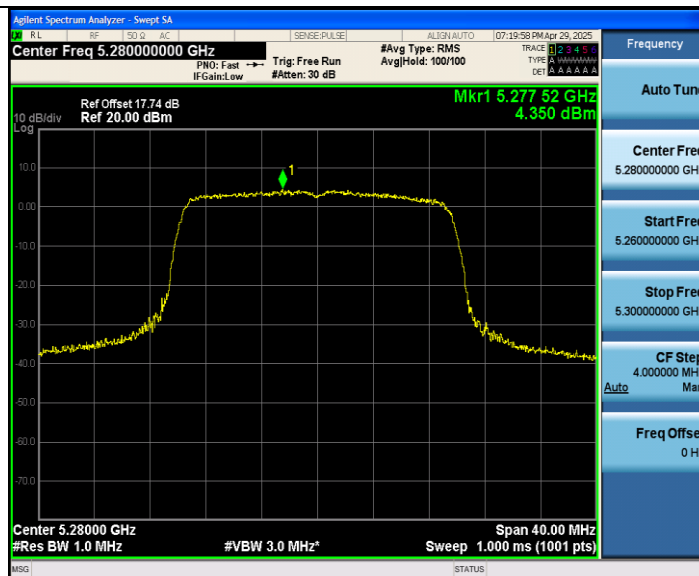
11AX20MIMO Ant2 5280
