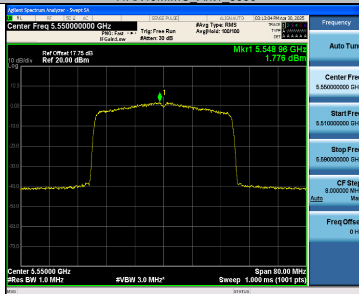
11AX40MIMO_Ant2_5550
