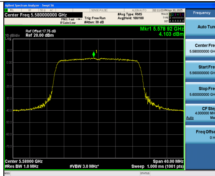
11AX20MIMO_Ant2_5580
