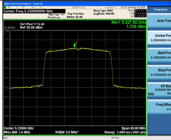
11AX40MIMO_Ant2_5230
