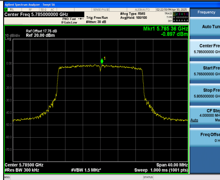
11AX20MIMO_Ant2_5785
