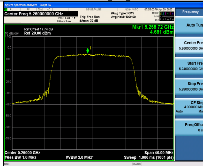
11AX20MIMO_Ant2_5260
