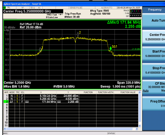
11AC160MIMO_Ant2_5250
