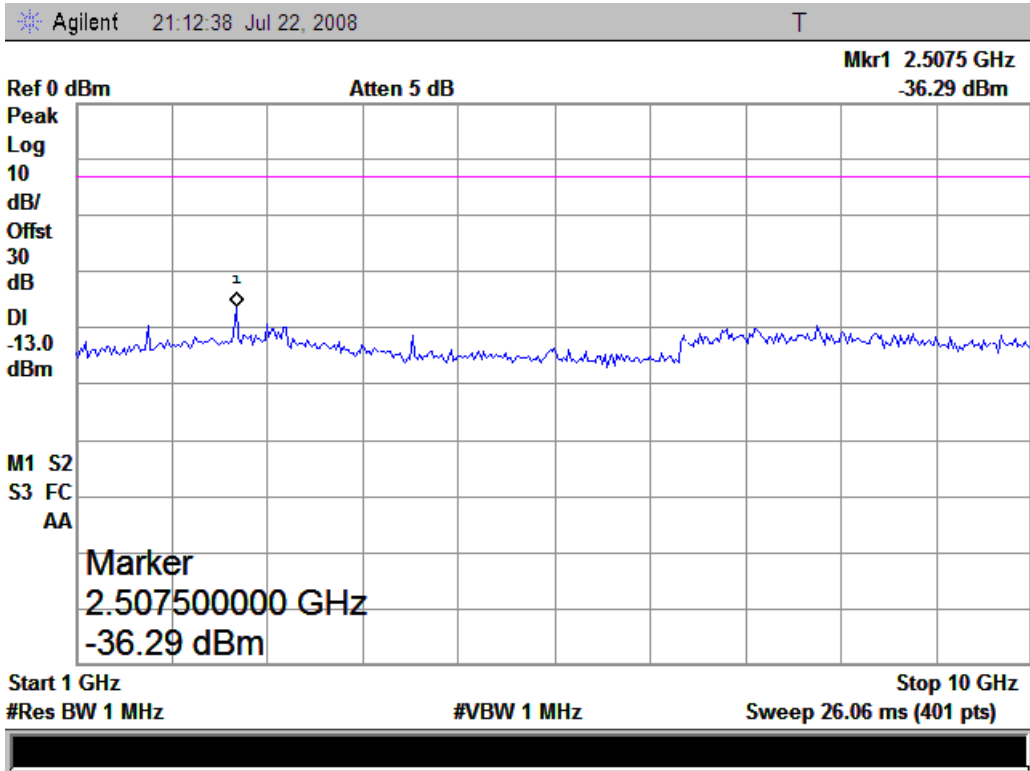
(1 GHz-10 GHz)
