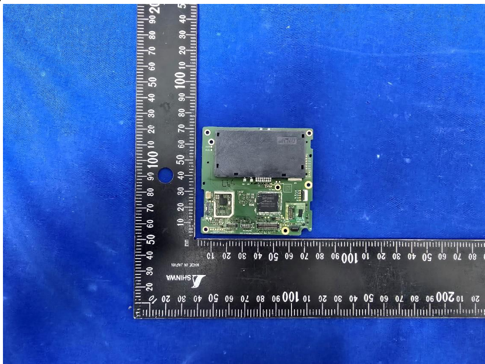
(18)EUT Photo
