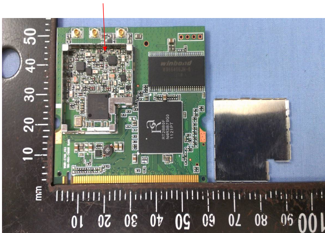
WLAN Module
