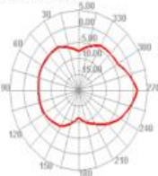
5250.000MHz H
