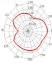
5350.000MHz E2
