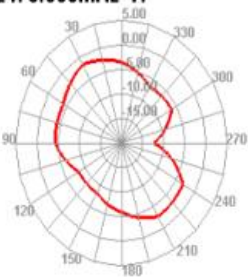
2475.000MHz E2
