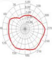
5150.000MHz E2
