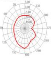
5150.000MHz E1
