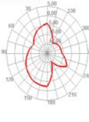
5350.000MHz E1
