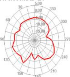
2475.000MHz E1
