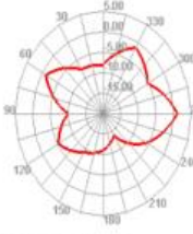
5350.000MHz E2
