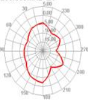
5250.000MHz E1
