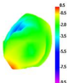
2475.000MHz E1
