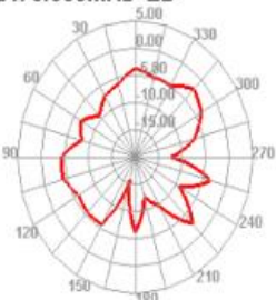
2475.000MHz E2
