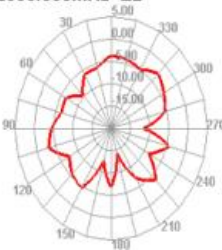
2500.000MHz E2
