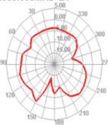
2500.000MHz E1
