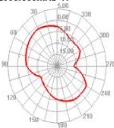
2500.000MHz H
