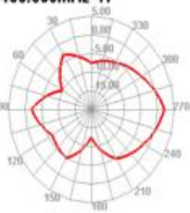
5150.000MHz E2
