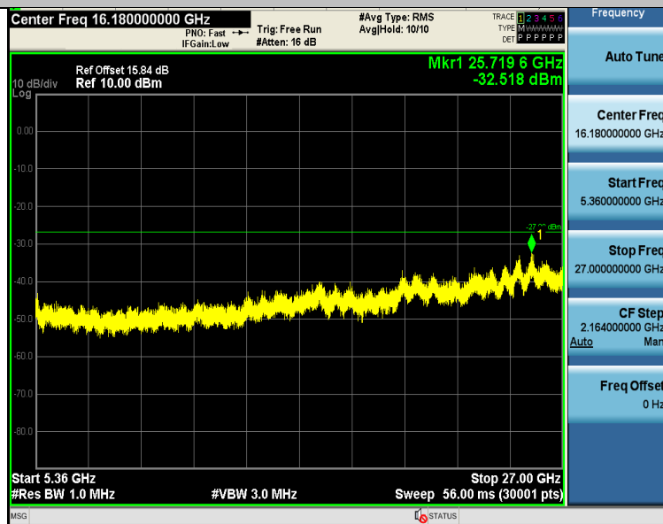
11A-Ant1-5200-5360~27000-PASS
