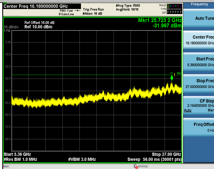
11A-Ant1-5240-5360~27000-PASS
