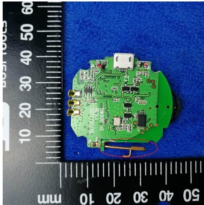
Antenna View(PP)
