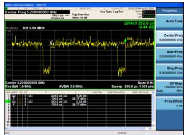
802.11ax(160MHz)
