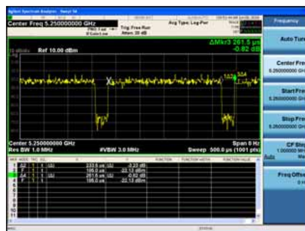
802.11ax(160MHz)
