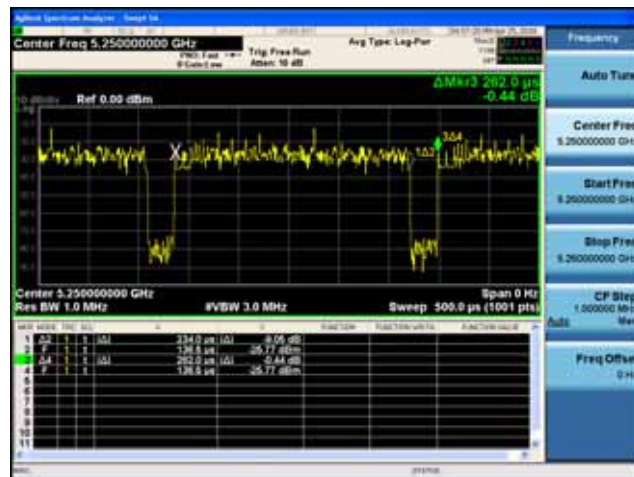
802.11ax(80MHz)
