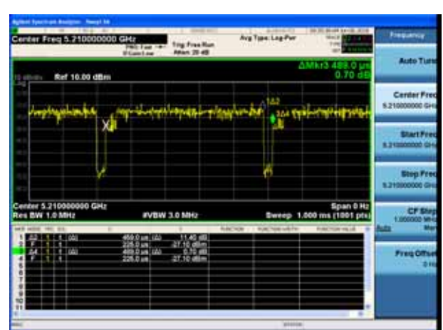
802.11ac(80MHz)
