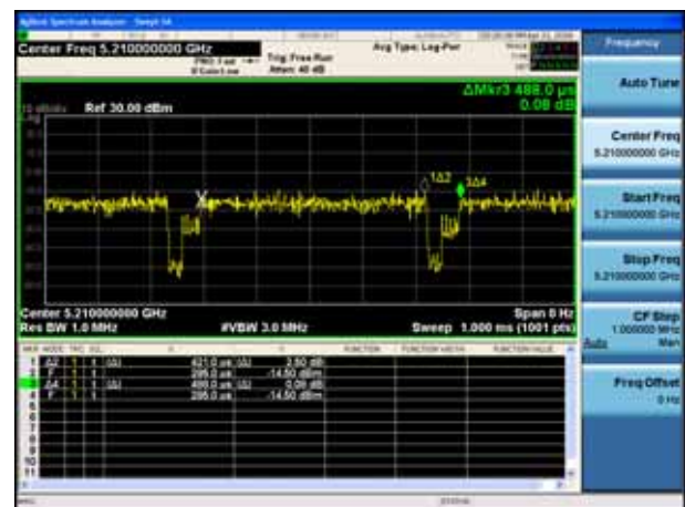
802.11ac(80MHz)
