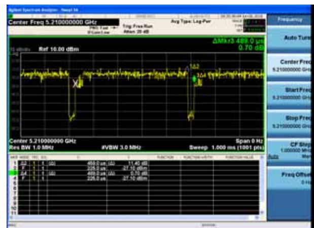
802.11ac(80MHz)
