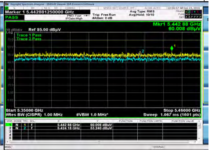
802.11ac-VHT 5290M(5350-5460MHz)
