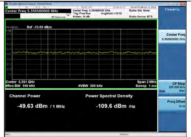
Band Edge -802.11a-5320M-chain3
