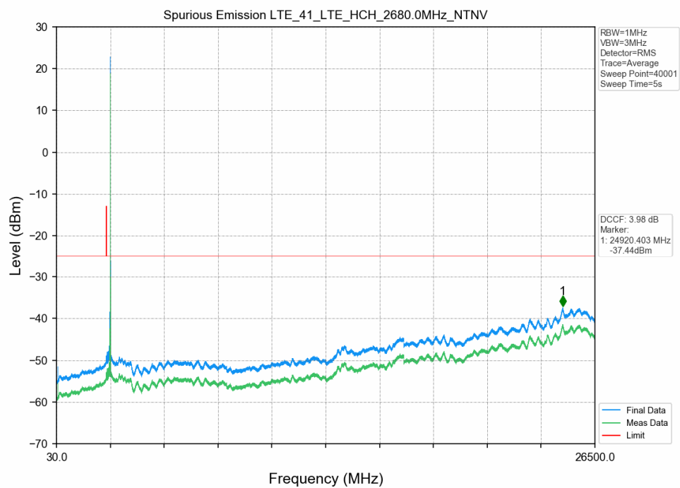
16QAM_20MHz
