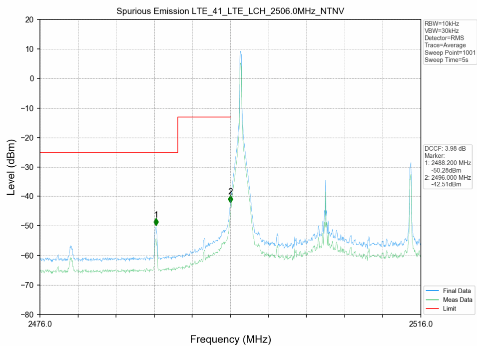
QPSK_20MHz
