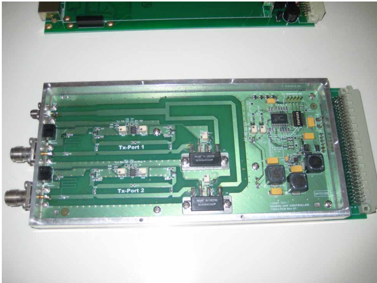
70003 UHF Controller
