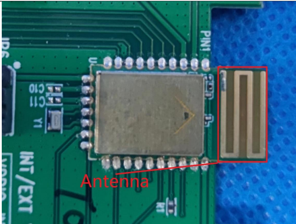
(8) EUT Photo - CYW20822-P4EPI040
