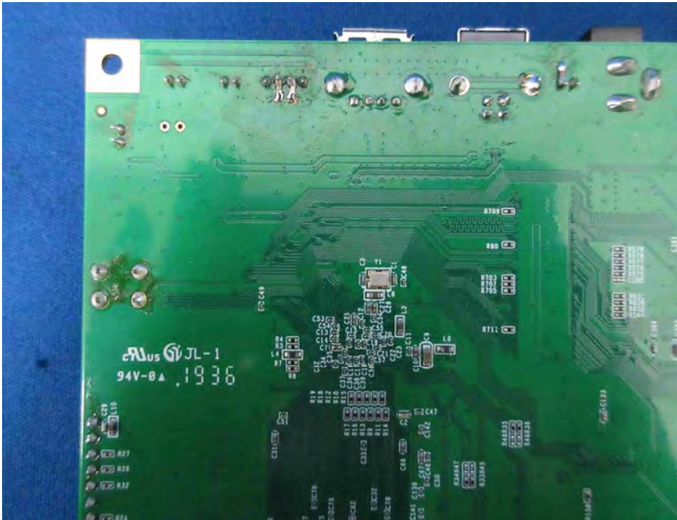
(46) EUT Photo
