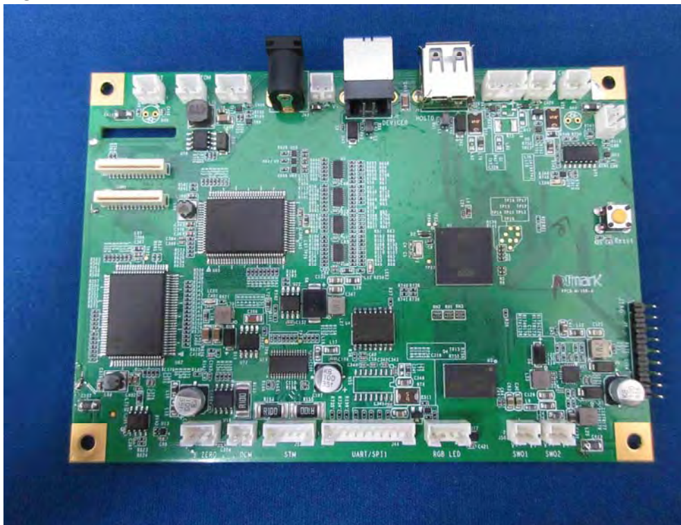
(44) EUT Photo
