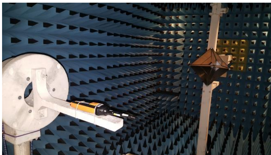
Fig. 1: Photo of DUT.
