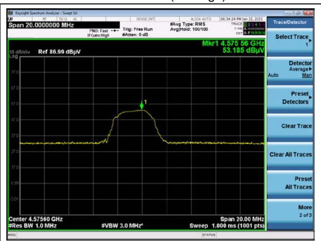
5 th harmonic (Average)
