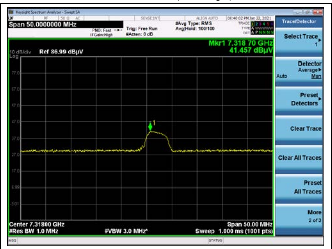
8 th harmonic (Average)
