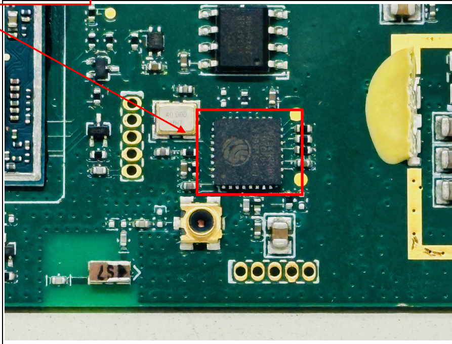
WLAN Module
