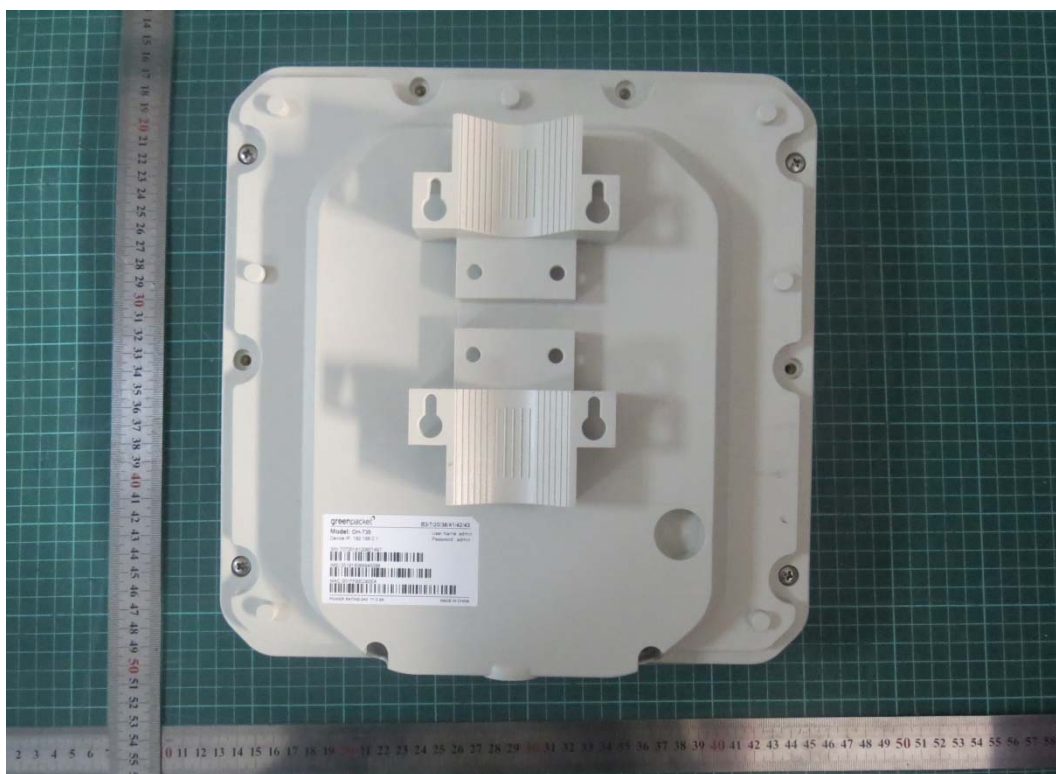
a: EUT
