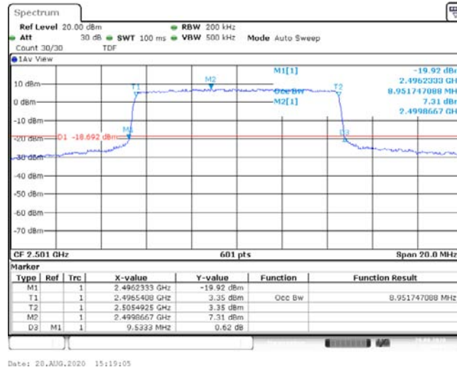
Band41-10MHz-QPSK-39700-50RB#0-8.952-9.533-PASS
