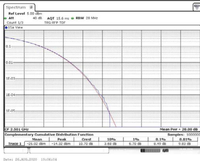
Band41-10MHz-QPSK-39700-50RB#0-8.49-13-PASS
