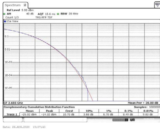
Band41-10MHz-QPSK-41540-50RB#0-8.49-13-PASS
