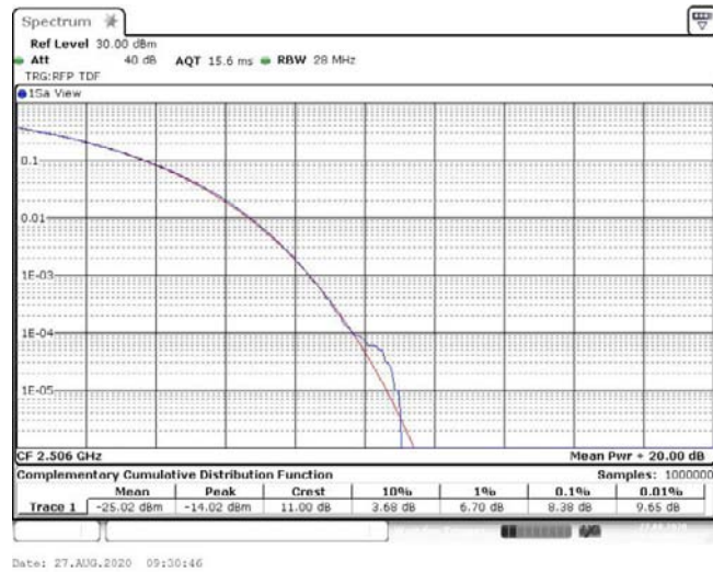
Band41-20MHz-QPSK-39750-1RB#0-8.38-13-PASS
