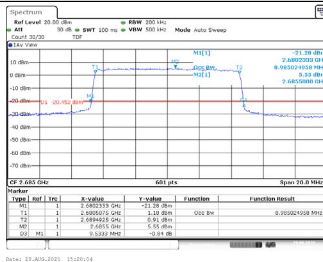
Band41-10MHz-QPSK-41540-50RB#0-8.985-9.533-PASS
