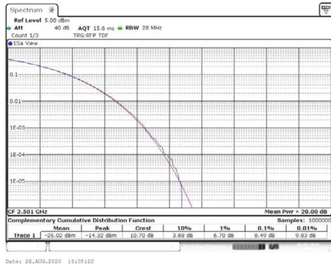
Band41-10MHz-QPSK-39700-1RB#0-8.49-13-PASS
