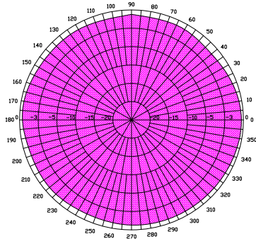
水平方向图
