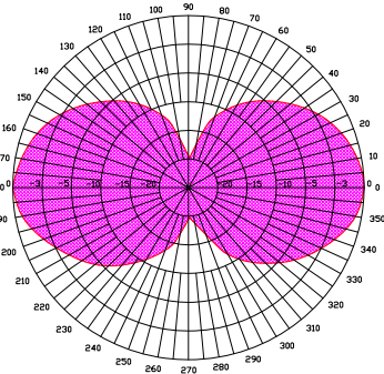
垂直方向图
