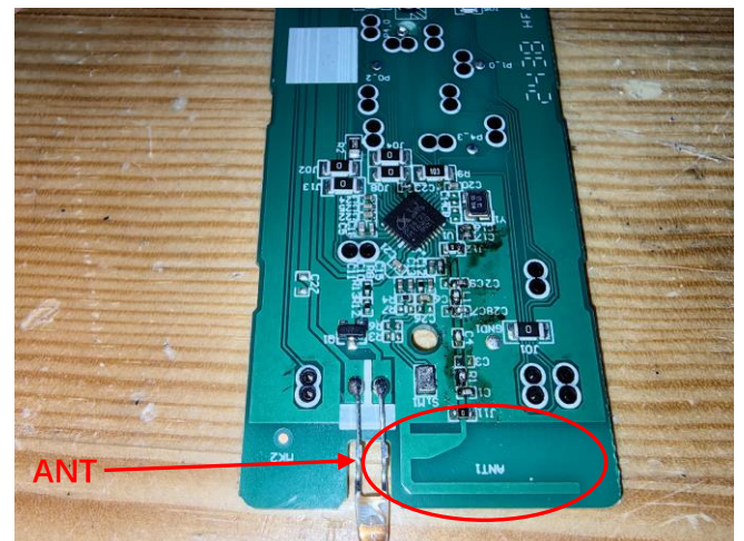
Antenna
