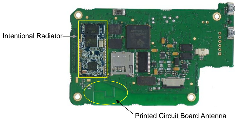
PCB Top
