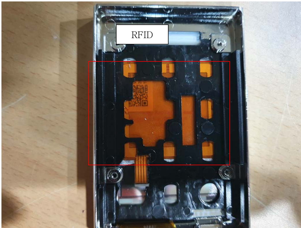
ANTENNA(2.4 GHz)
