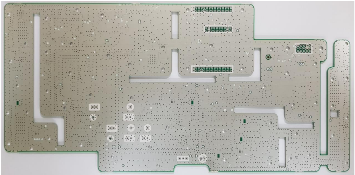
RX PCB Bottom
