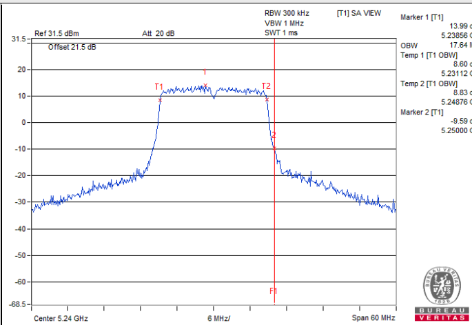
802.11ac (VHT20) / Chain 1 : CH 48
