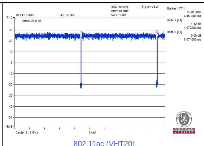
802.11ac (VHT20)
