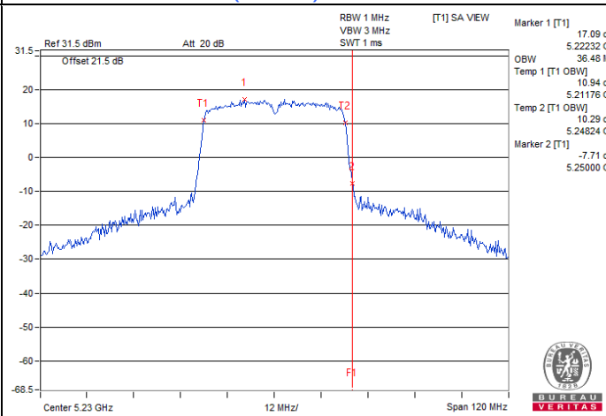
802.11ac (VHT40) / Chain 1 : CH 46
