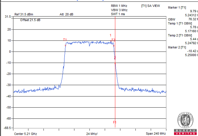
802.11ac (VHT80) / Chain 1 : CH 42
