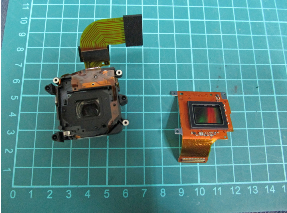
(72) EUT Photo
