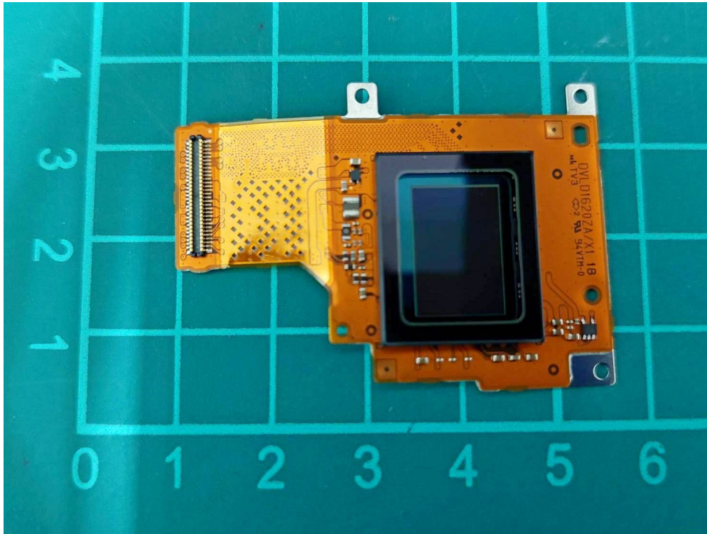
(75) EUT Photo
