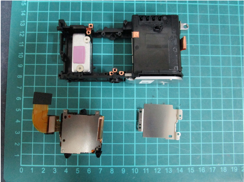
(71) EUT Photo
