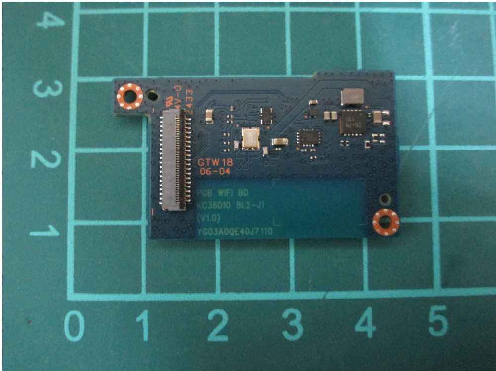
(69) EUT Photo
