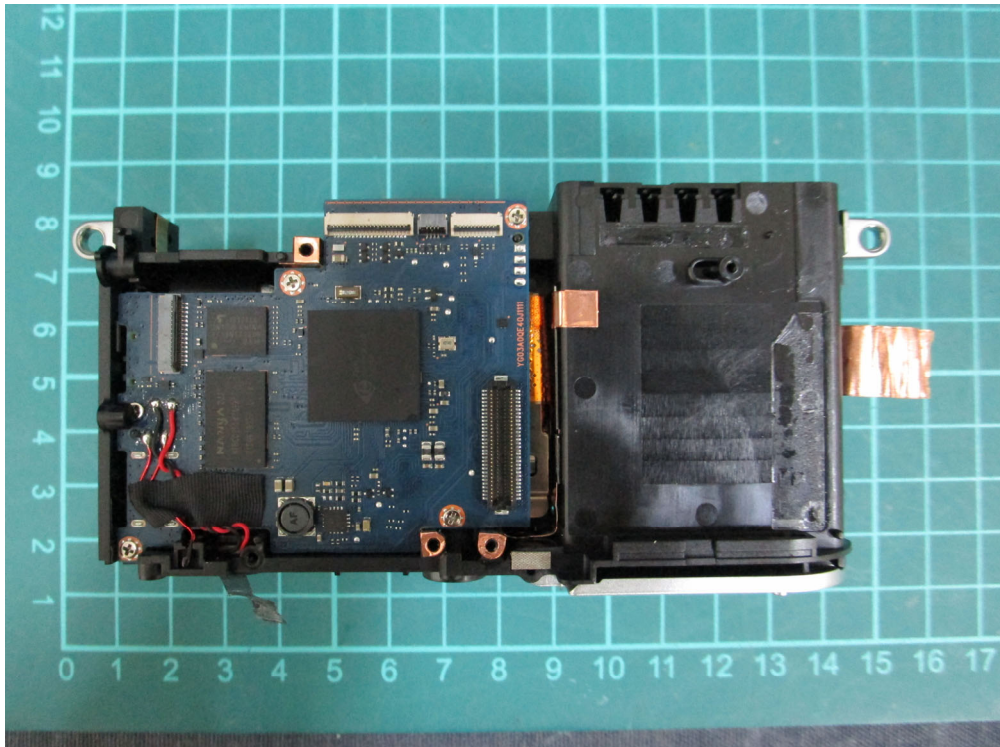
(46) EUT Photo
