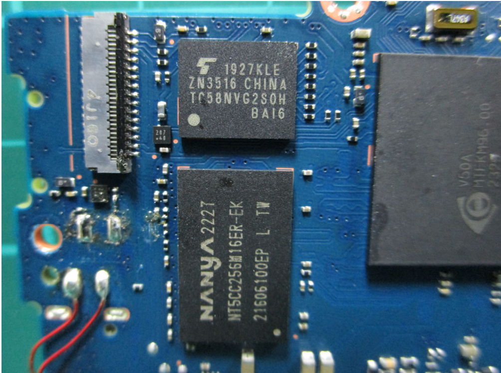
(59) EUT Photo
