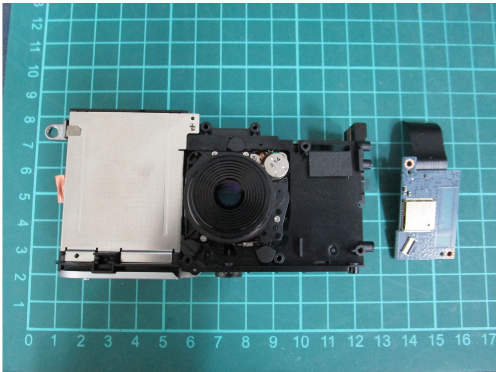
(62) EUT Photo
