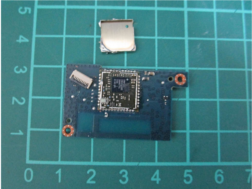
(64) EUT Photo
