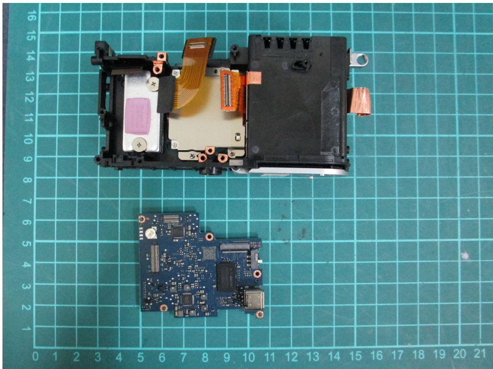
(52) EUT Photo
