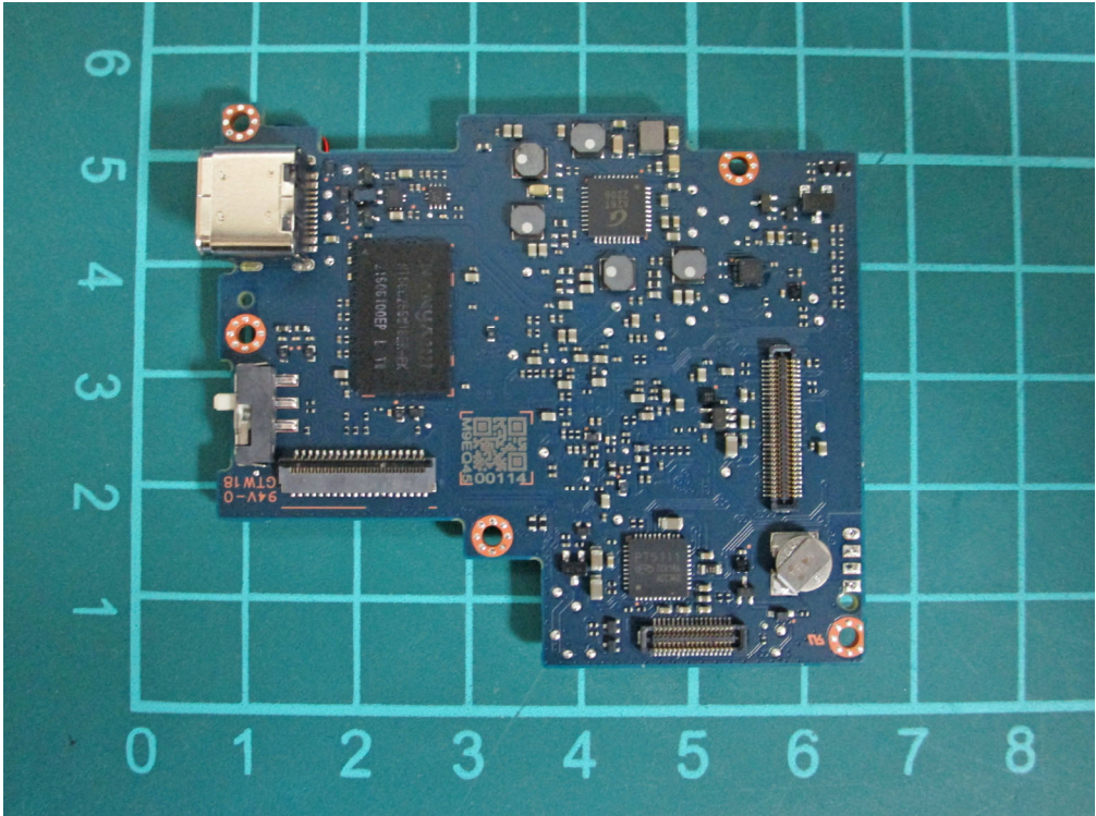
(53) EUT Photo
