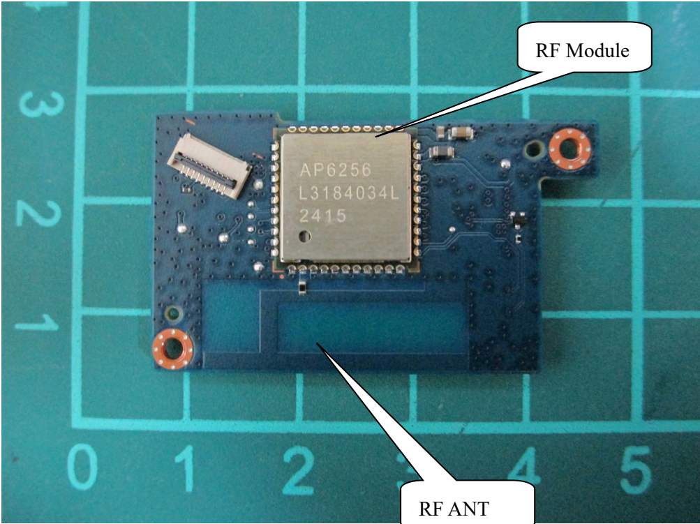
(63) EUT Photo
