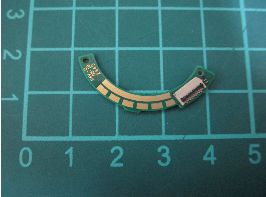
(50) EUT Photo
