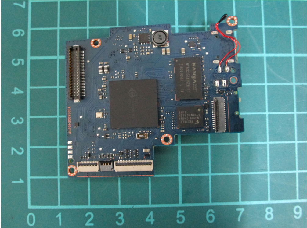
(54) EUT Photo
