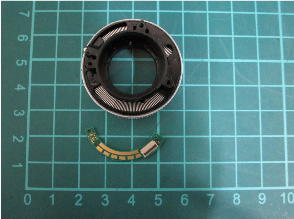
(49) EUT Photo
