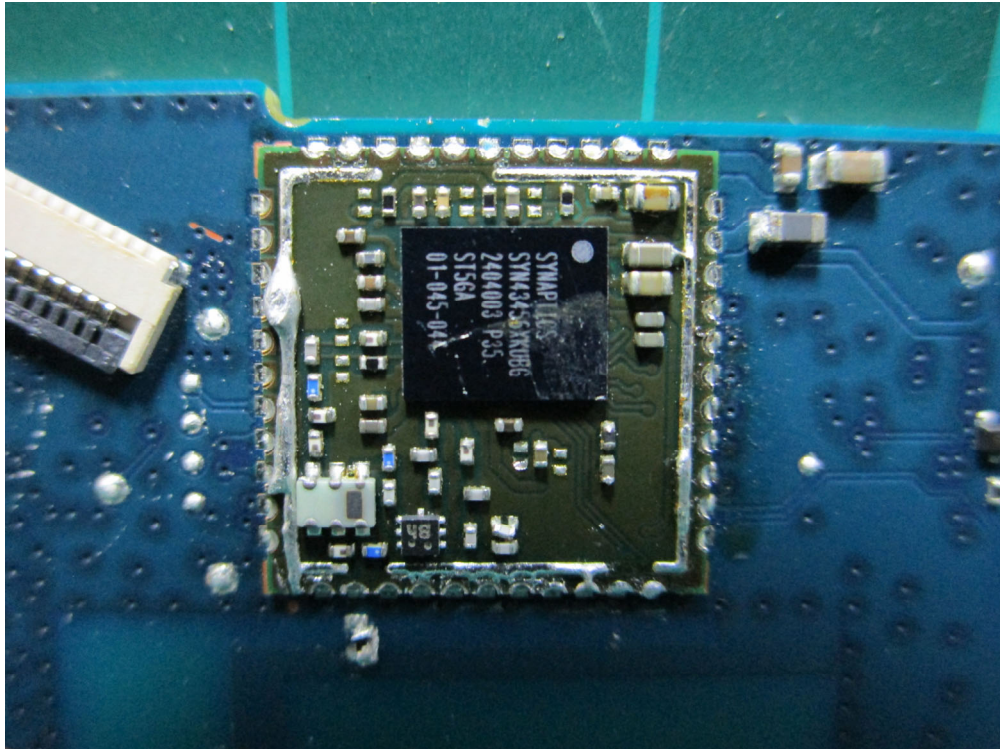
(65) EUT Photo
