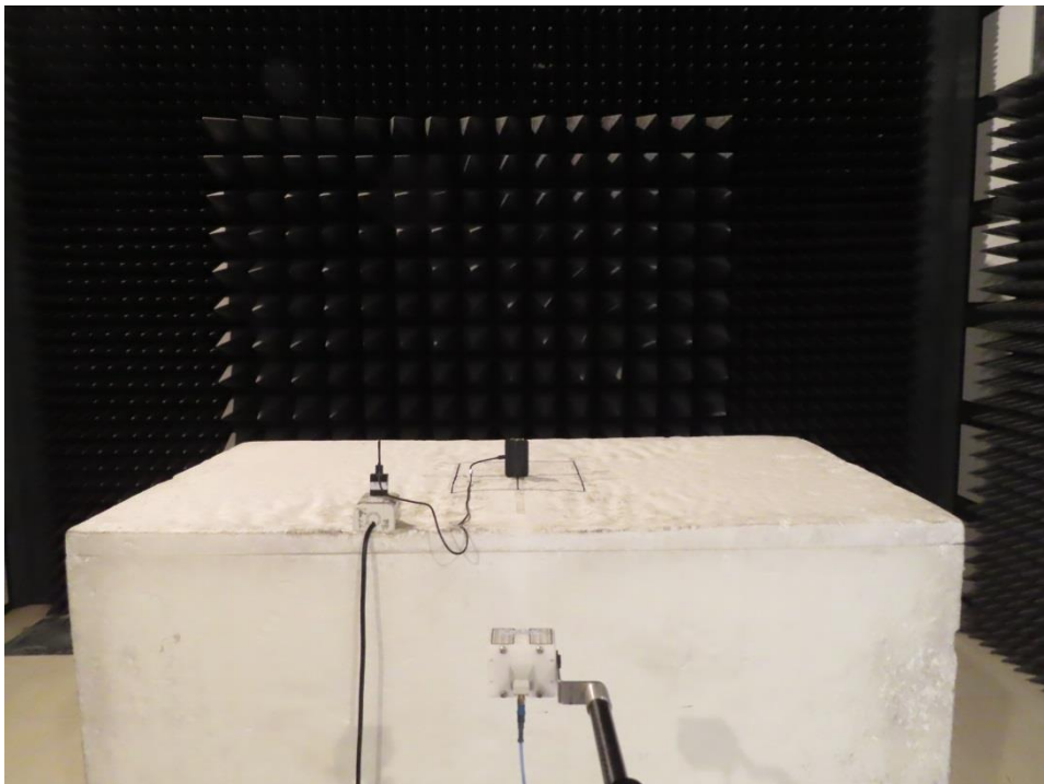
18GHz ~ 40GHz
