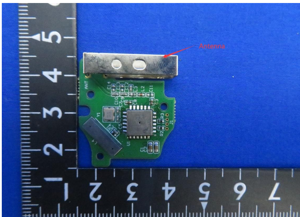
(4) EUT Photo
