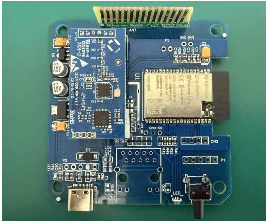
DD7006M Internal: Top
