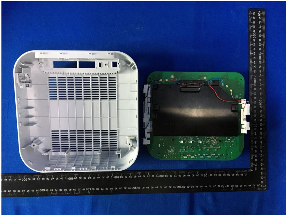
(3) EUT Photo (EVT2 Sample)
