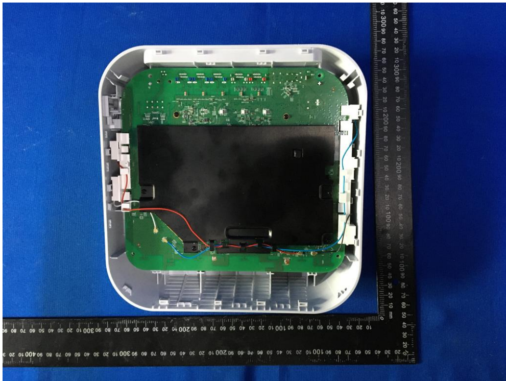
(2) EUT Photo (EVT2 Sample)
