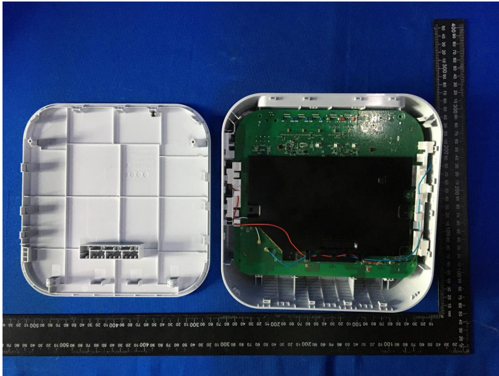
(1) EUT Photo (EVT2 Sample)
