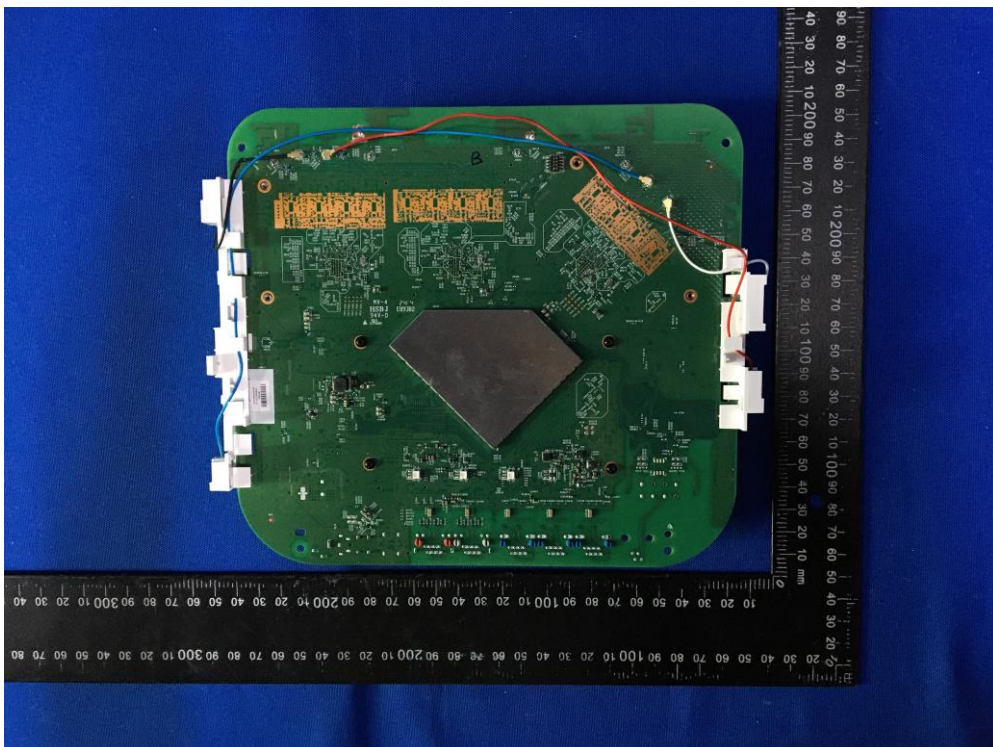
(8) EUT Photo (EVT2 Sample)
