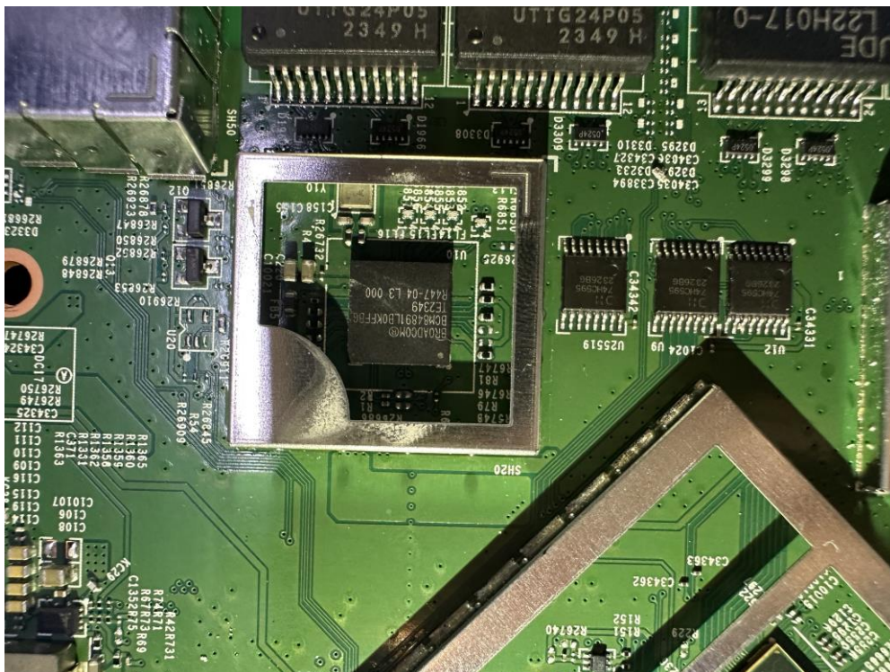
(14) EUT Photo (EVT2 Sample)
