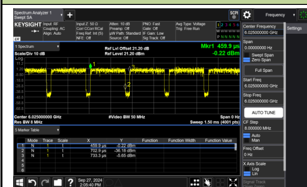
802.11be-EHT40
