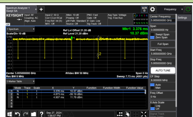
802.11be-EHT80
