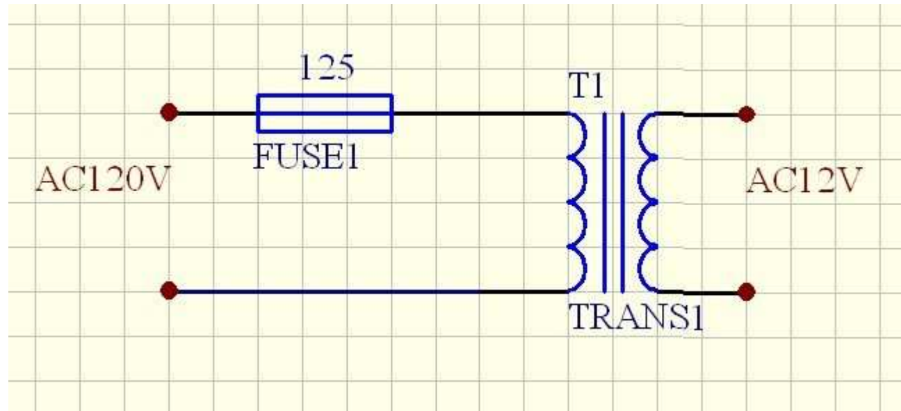
变压器电路图
