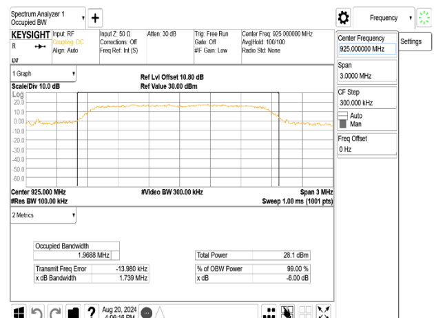
OBW_OFDM_2M_HighCH-925
