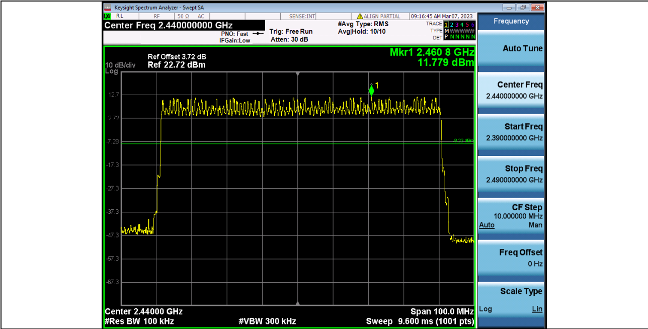
2_Band Edge (Hopping) NVNT_ANT1_2-DH5_Hopping
