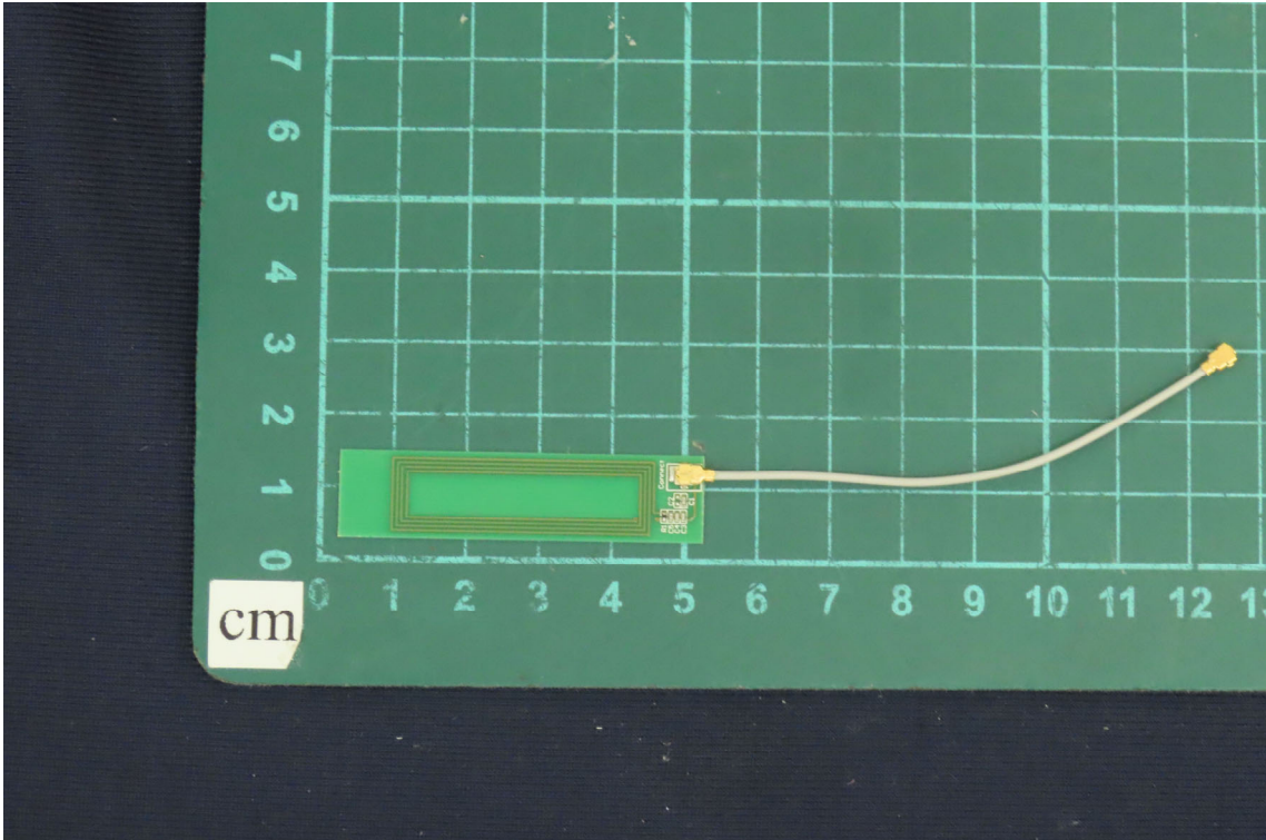
(9) EUT Photo
