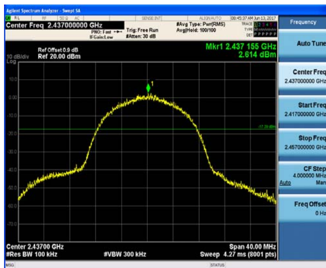
802.11b CH06
