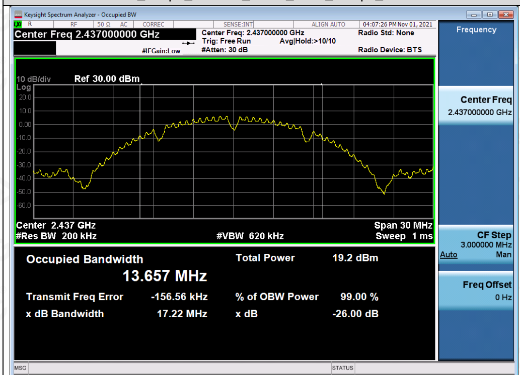
Test_Graph_802.11b_ANT1_2437_1Mbps_OBW
