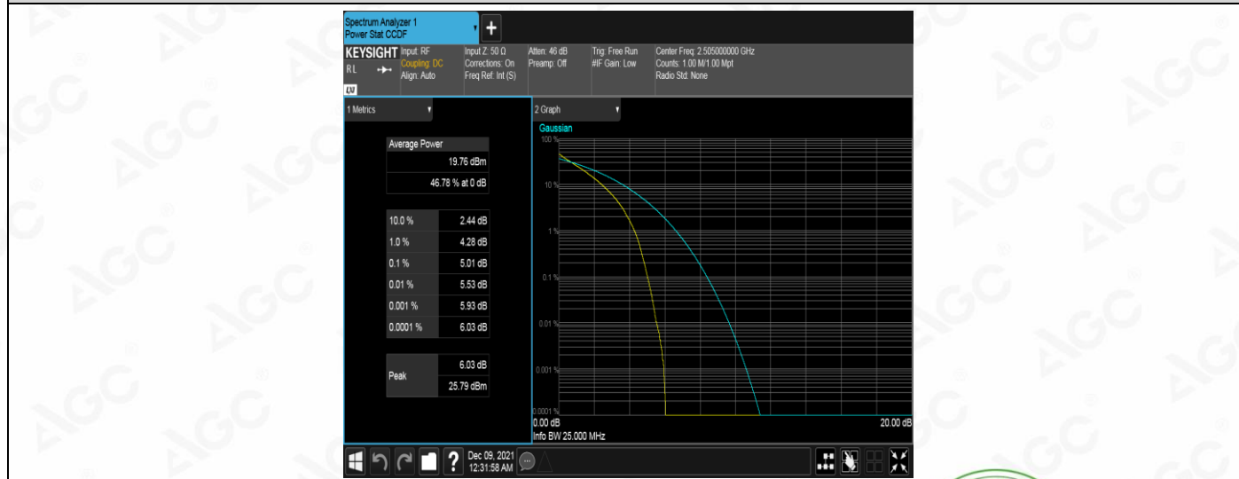
Band7-10MHz-QPSK-20800-50RB#0
