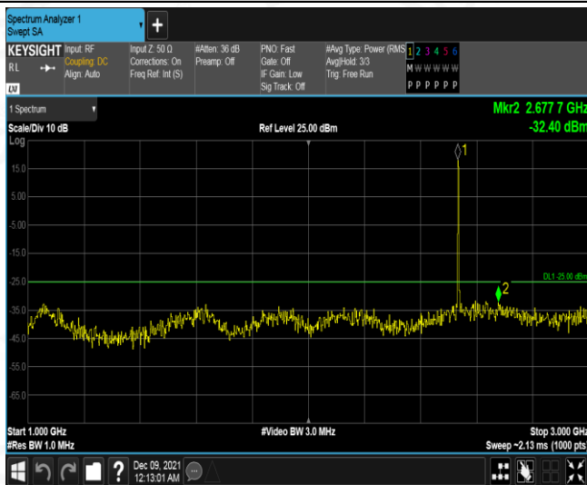
Band7-5MHz-QPSK-21100-1RB#0-Range2:1000~3000MHz
